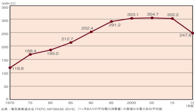
一世帯あたりの電力消費量の推移
